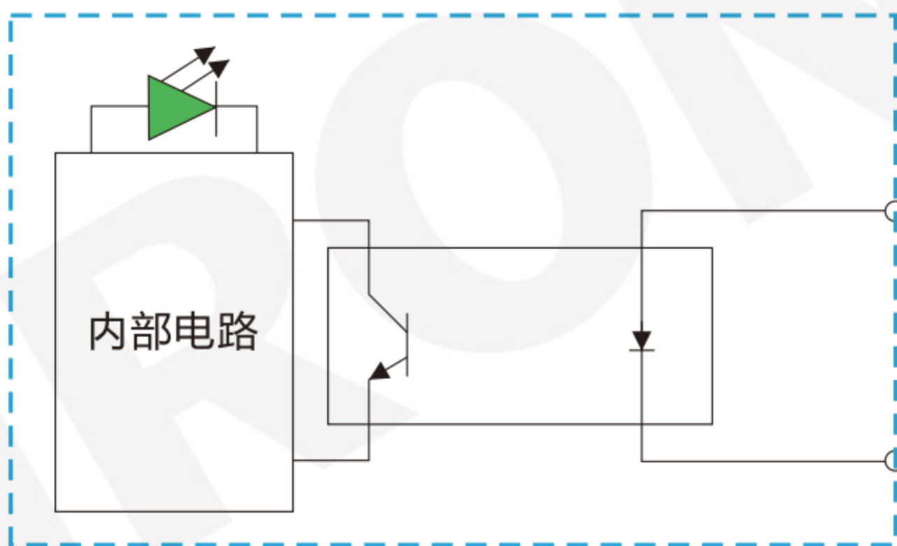
输入模组内部电气方框图
