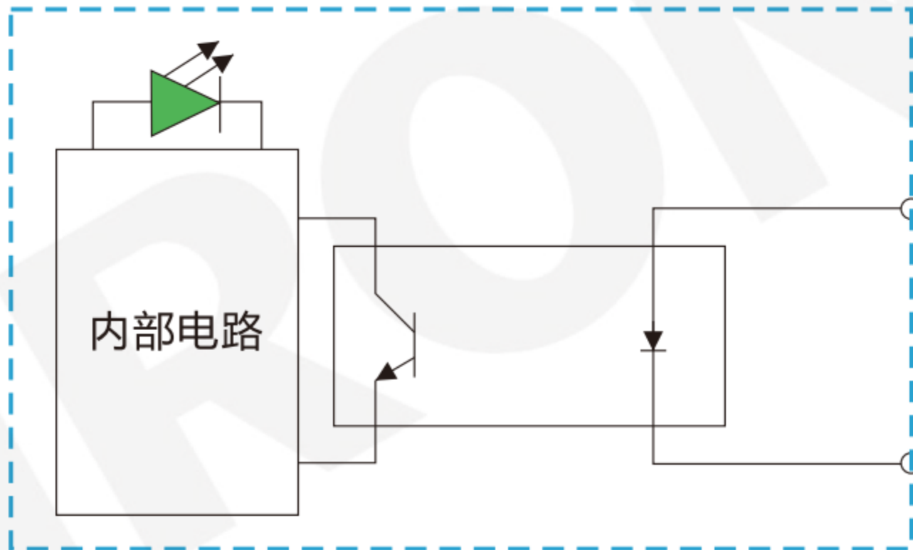
输入模組内部电气方框图
