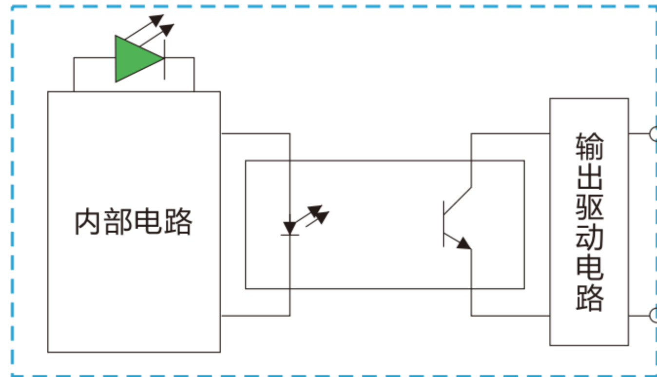
输出模組电气隔离方框图
